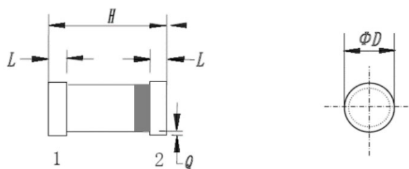
图 4 DO-213AB 外形尺寸
