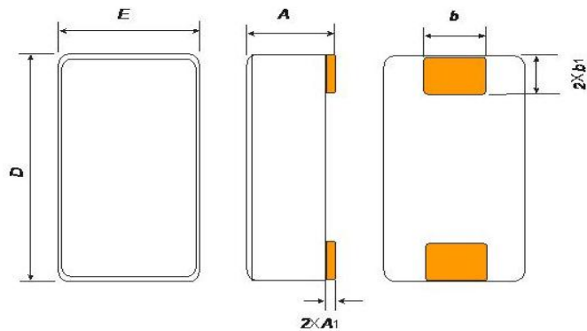
图 6 SMD-0.05 外形尺寸
