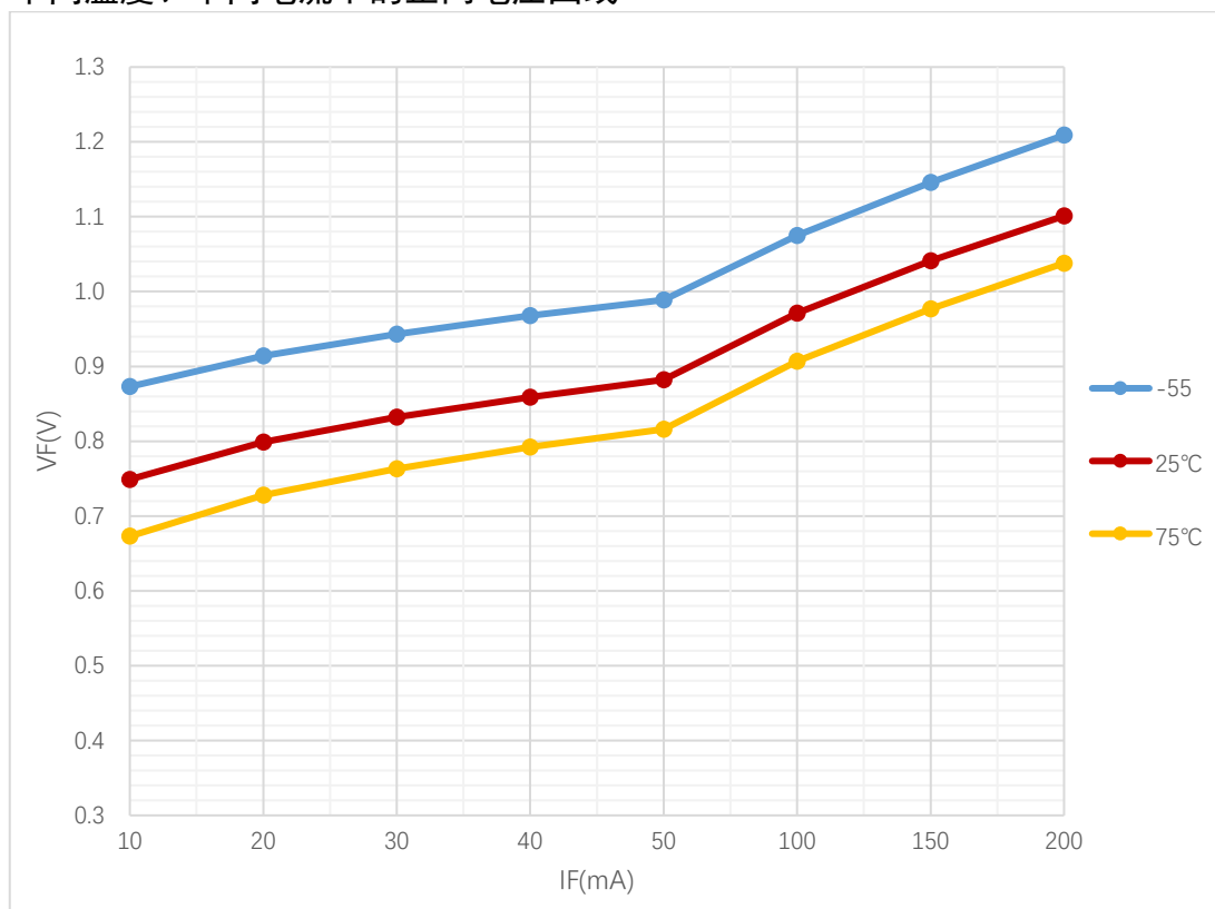
图 2 V_F — I_F 特性曲线
