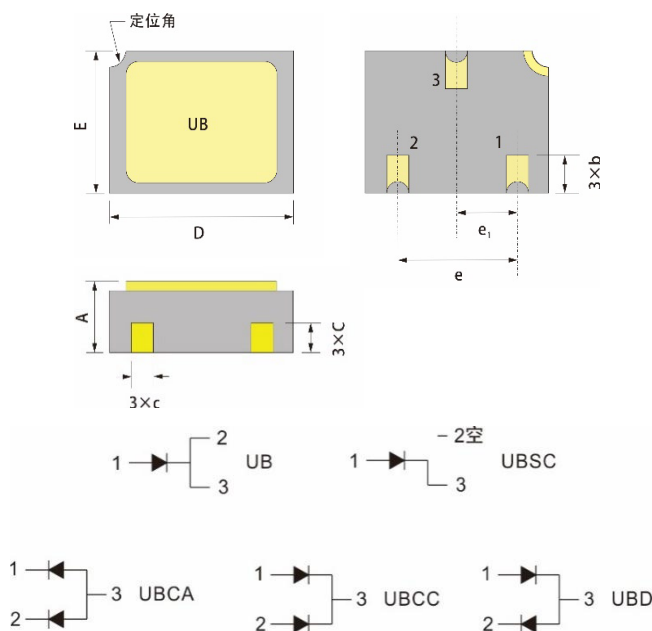
图 6 UB 外形尺寸
