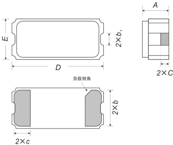
图 7 UC 外形尺寸
