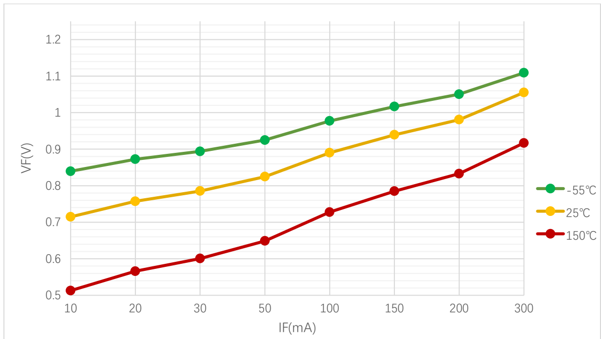
图 2 V_F - I_F 特性曲线
