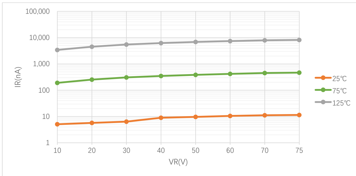
图 1 I_R - V_R 特性曲线
