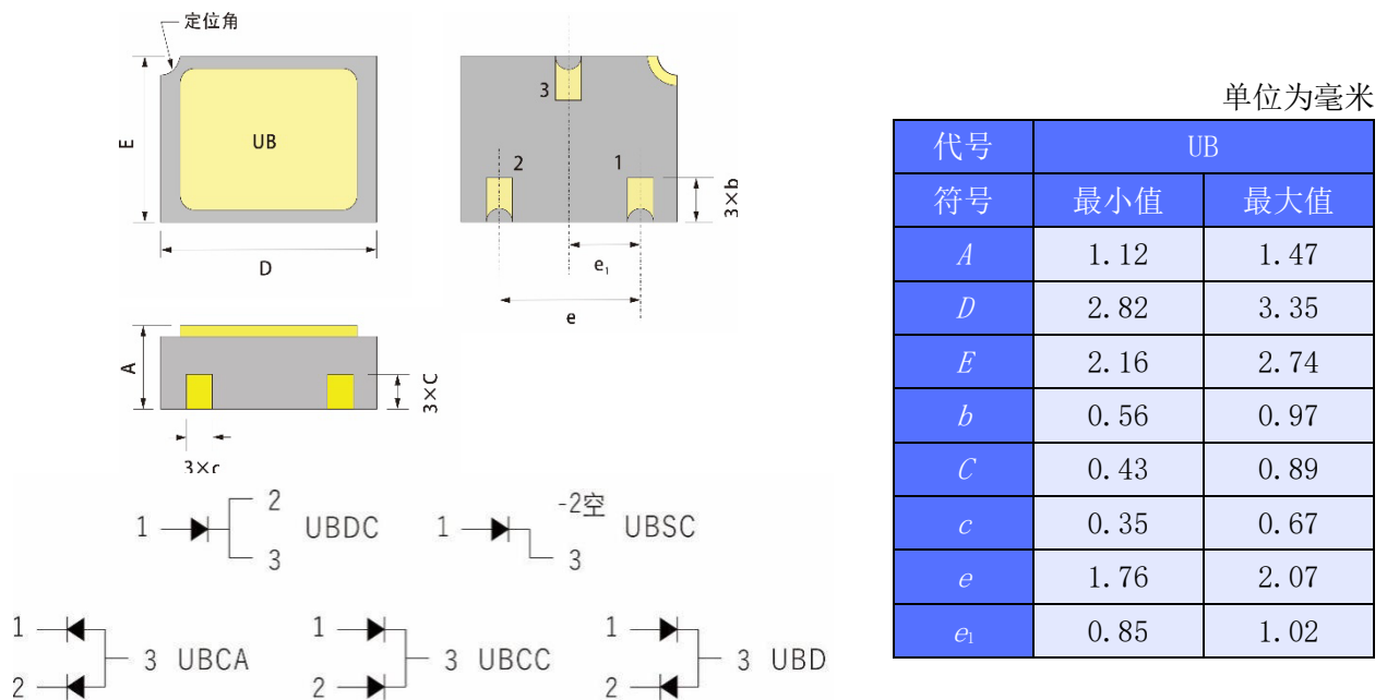
图 6 UB 外形尺寸
