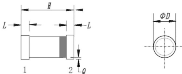
图 4 D2-05A 外形尺寸
