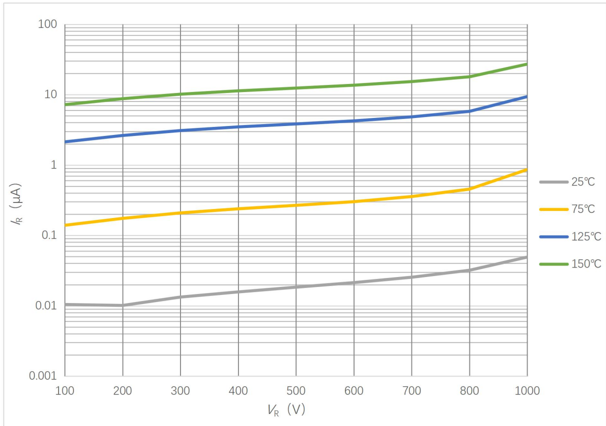
图1 I_R - V_R 特性曲线
