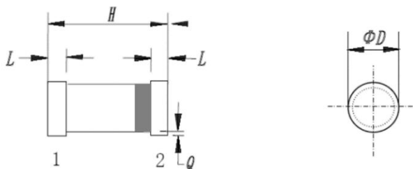
图 4 D2-05A 外形尺寸
