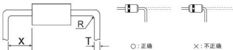
图 6 引线成型后示意图
