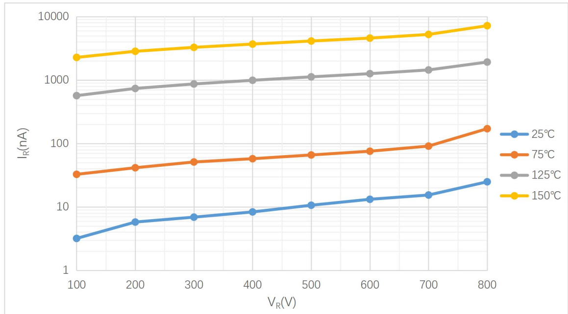
图 1 I_R — V_R 特性曲线
