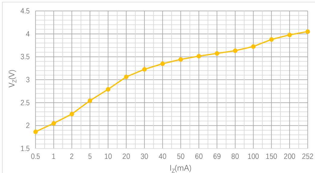
图 1 V_z-I_z 特性曲线
