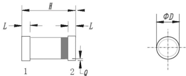
图 4 D0-213AB 外形尺寸
