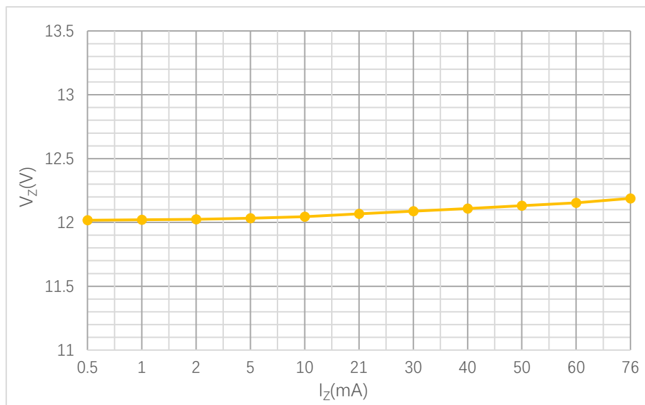
图 1 V_Z-I_Z 特性曲线
