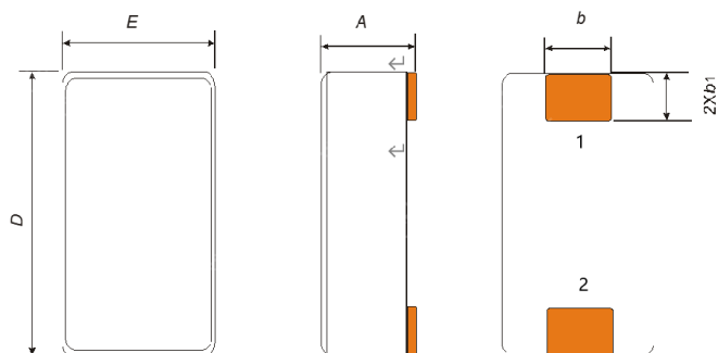
图 5 SMD-0.1 外形尺寸
