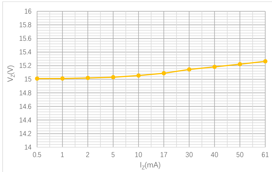
图 1 V_Z-I_Z 特性曲线
