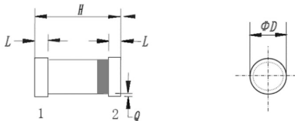
图 3 D2-05A 外形尺寸
