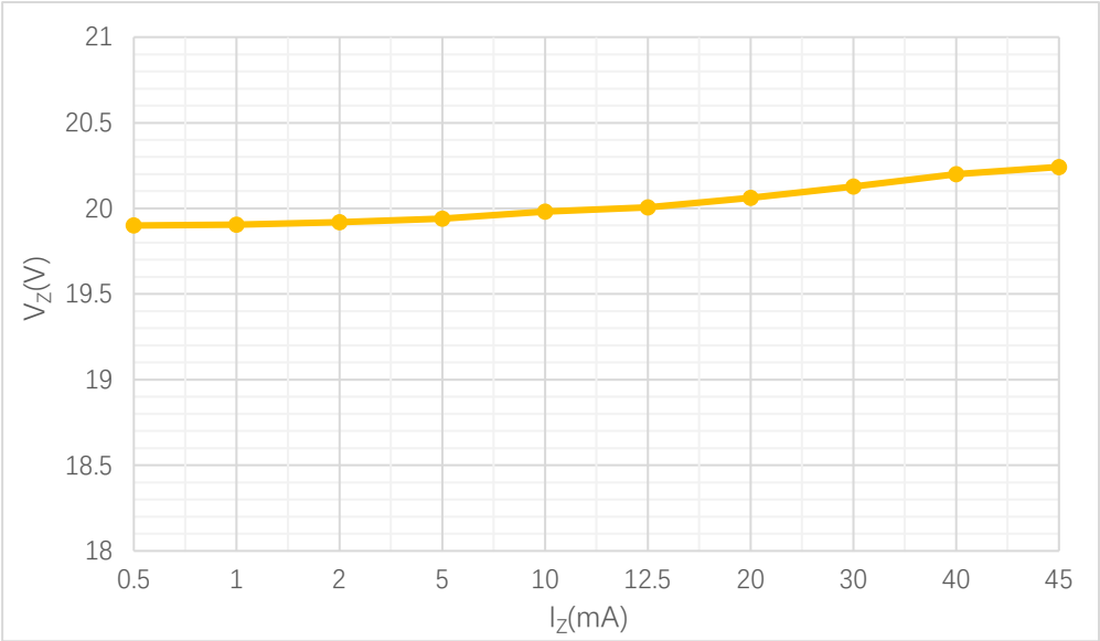
图 1 V_Z - I_Z 特性曲线
