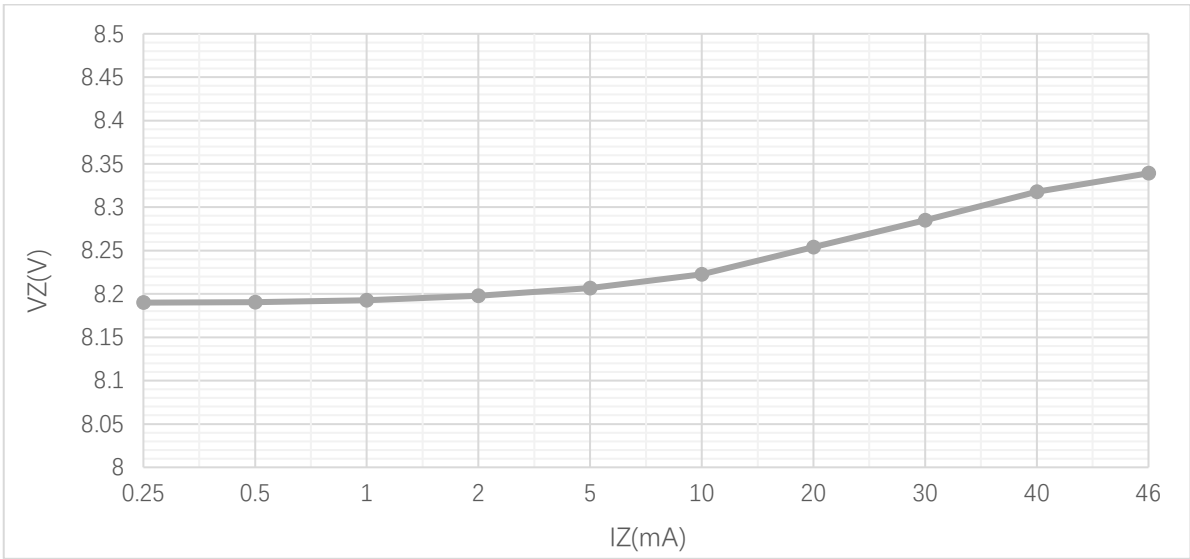
图 1 V_Z — I_Z 特性曲线
