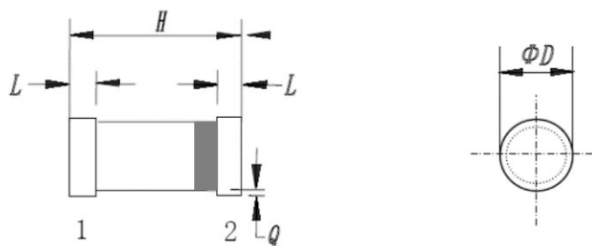
图 2 D2-02A 外形尺寸
