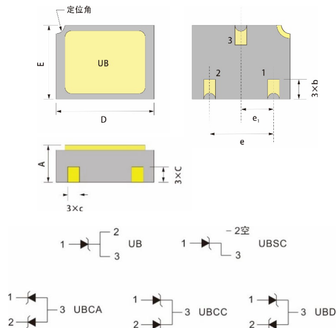
图 4 D0-213AA 外形尺寸
