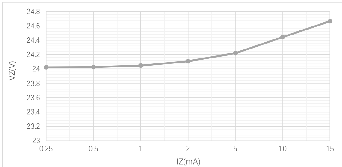
图 1 V_Z-I_Z 特性曲线
