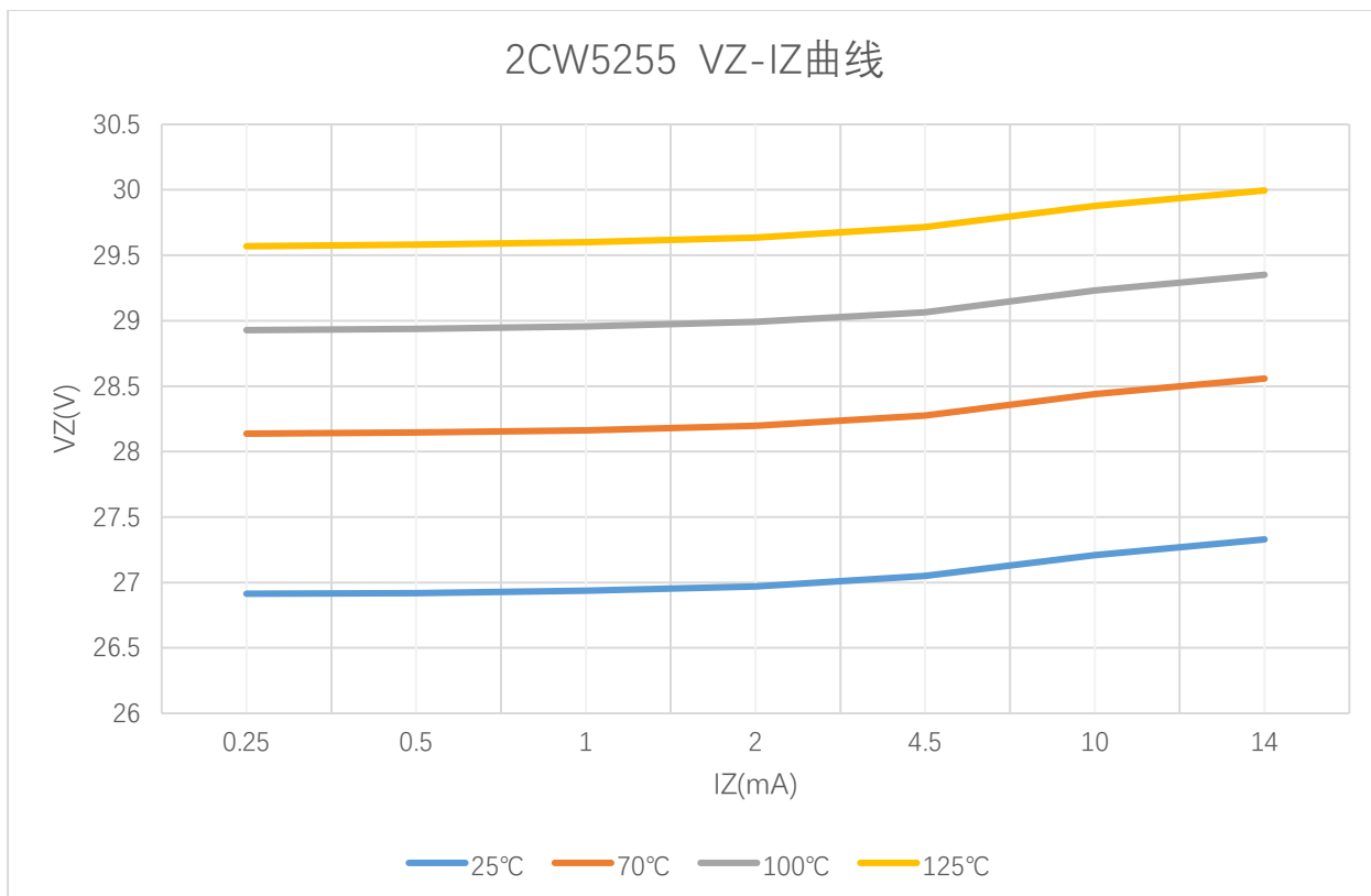
图 1 V_Z-I_Z 特性曲线
