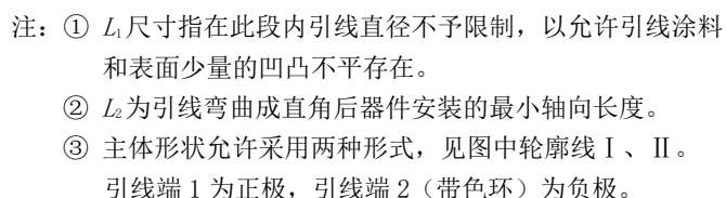
图 3 D2-02A 外形尺寸
