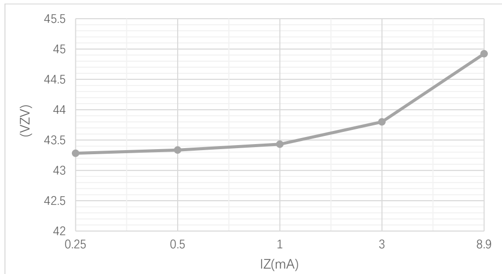
图 1 V_Z-I_Z 特性曲线
