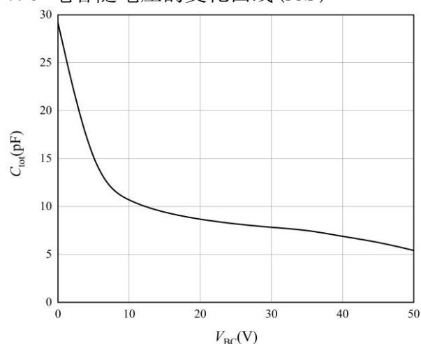
图 8 电容-电压特性曲线
