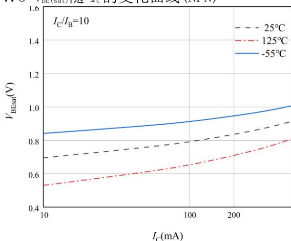
图 5 BE 端饱和压降特性曲线
