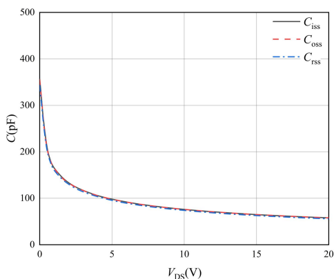
图 5 C-V_{DS} 特性曲线
