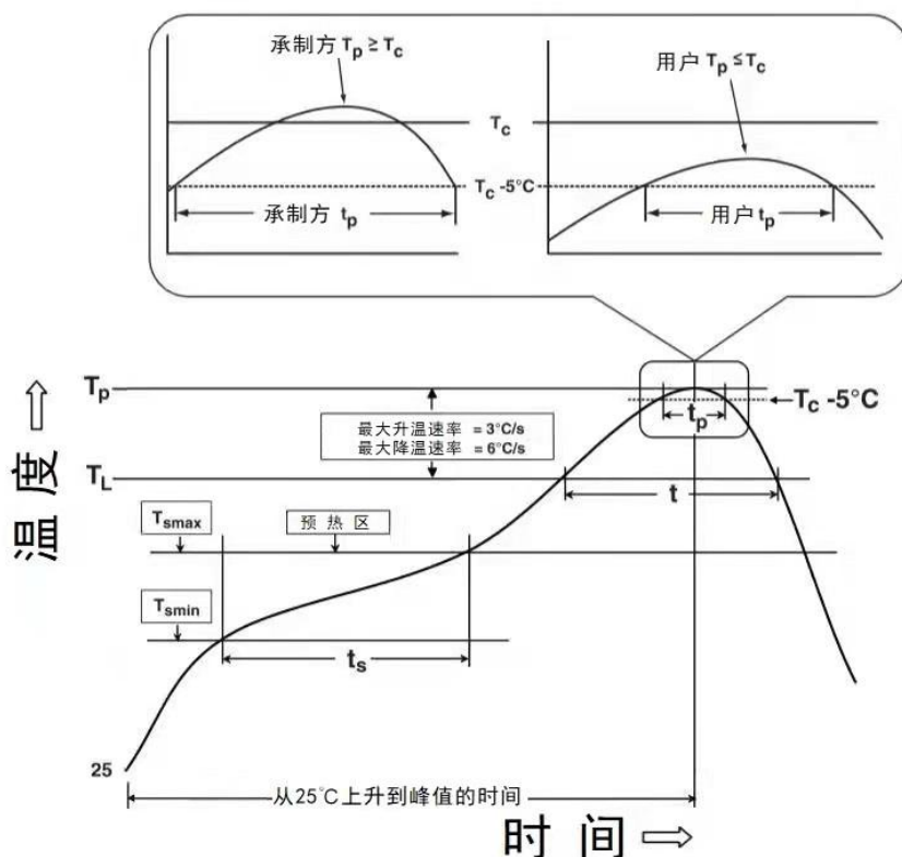
图 4 回流温度-时间分布图
