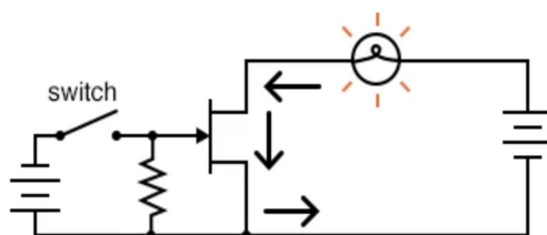
图 2 结型场效应管开关电路
