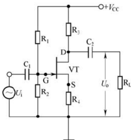
图 3 结型场效应管放大电路
