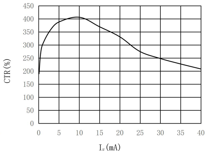
图2 I_F \sim \text{CTR} 关系曲线
