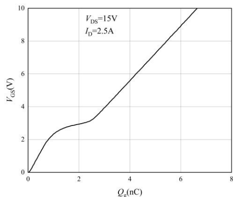
图 4 NMOS- V_{GS} - Q_g 特性曲线
