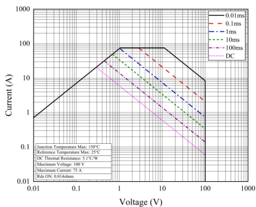
图 6 安全工作区曲线
