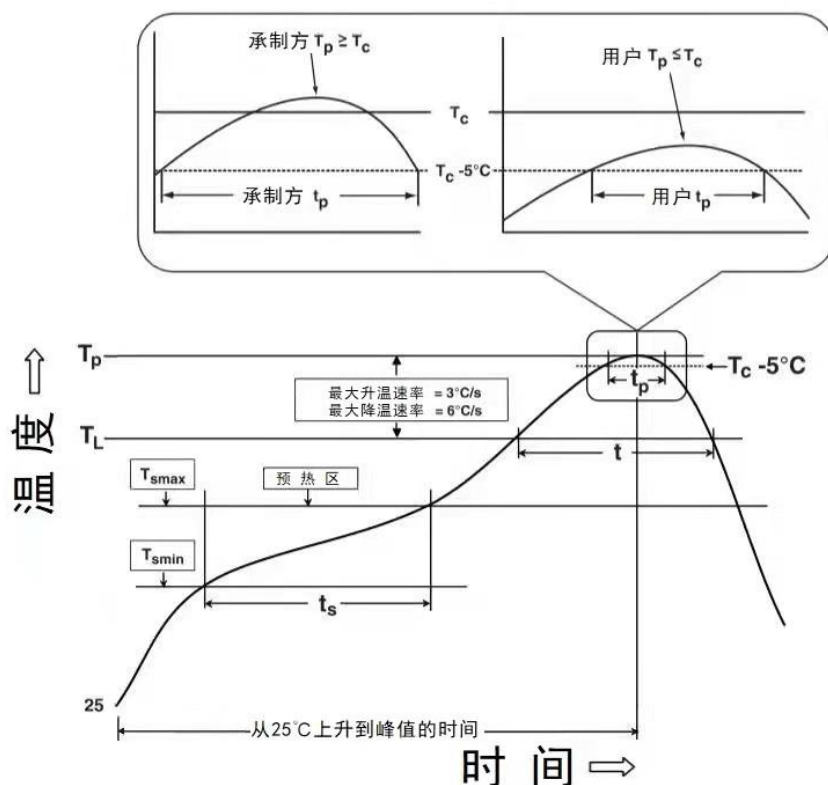
图 10 回流温度-时间分布图
