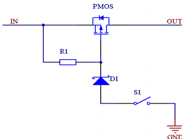
图 8 典型开关电路
