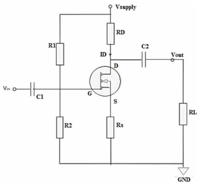
图 9 典型放大电路
