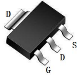
SOT-223
