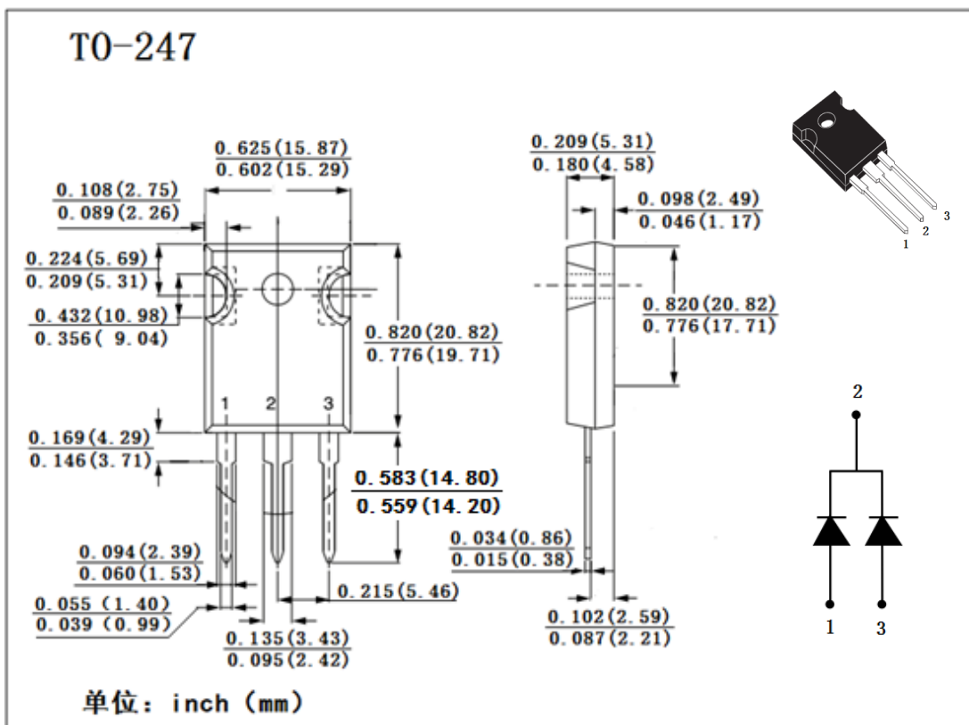
T0-247AB 封装外形图:
