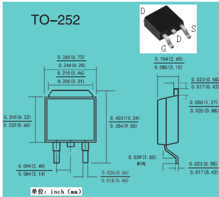
TO-252 封装外形图：
