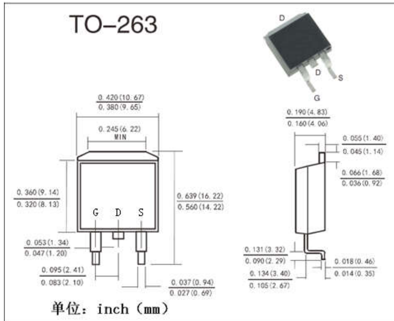
TO-263 封装外形图：
