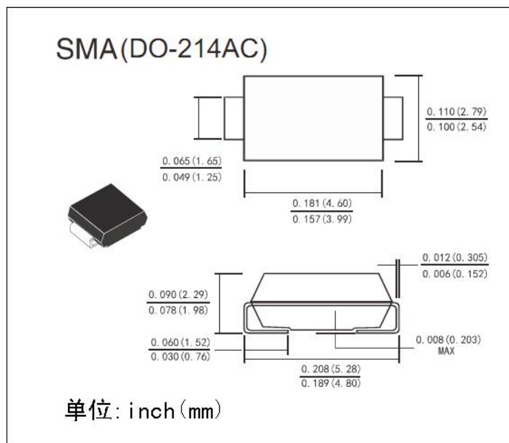
SMA 封装外形图: inch (mm)
