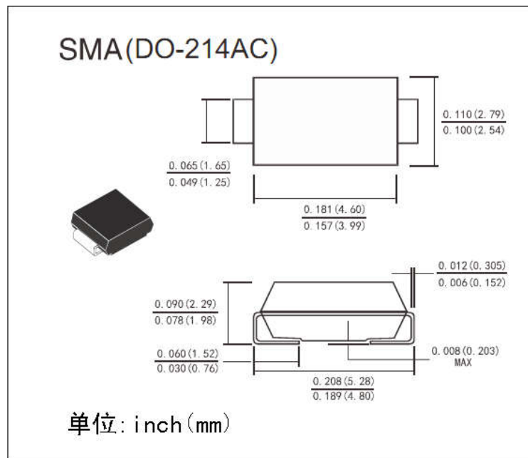
SMA 封装外形图: inch (mm)
