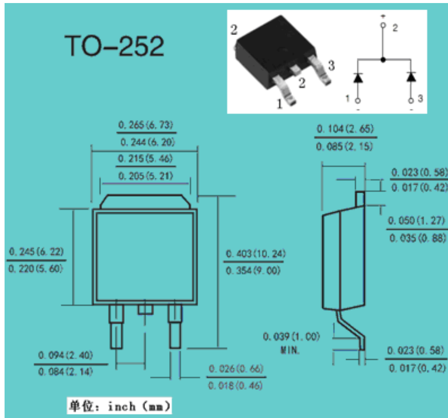
T0-252 封装外形图:
