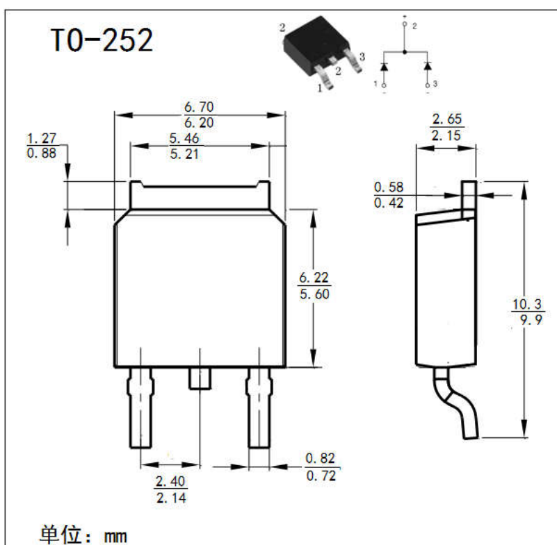
T0-252 封装外形图:
