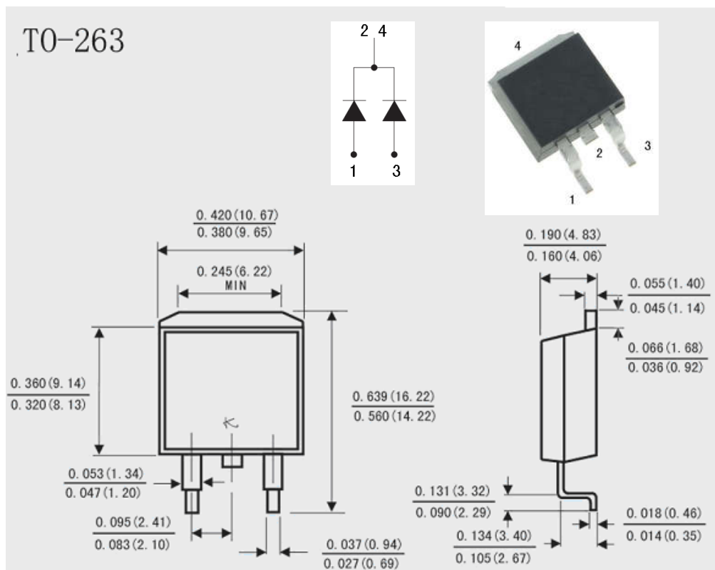
T0-263 封装外形图:
