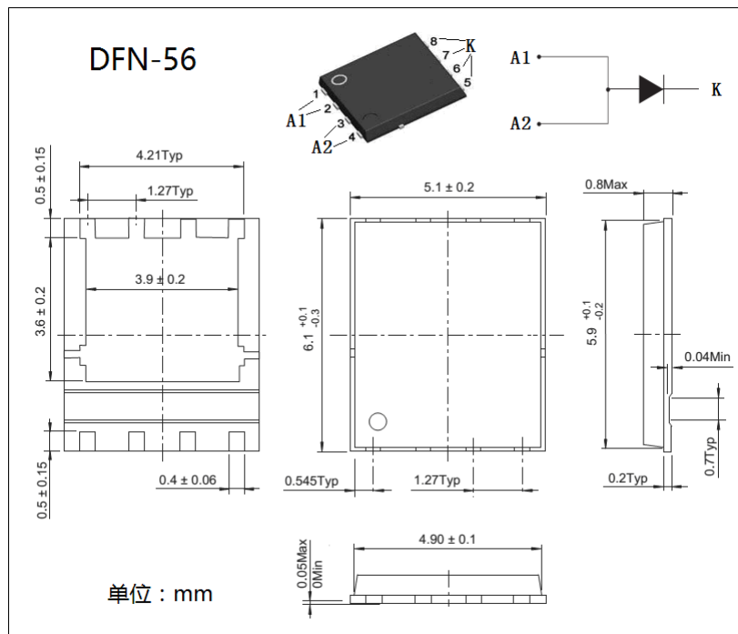
DFN-56 封装外形图:
