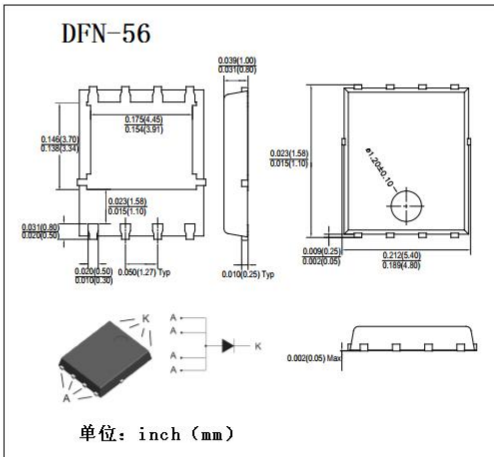
DFN-56 封装外形图:
