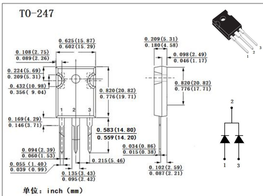
T0-247 封装外形图:
