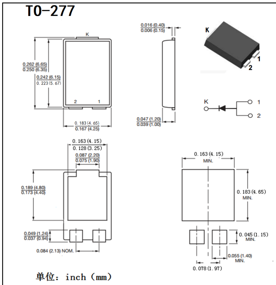
T0-277 封装外形图:
