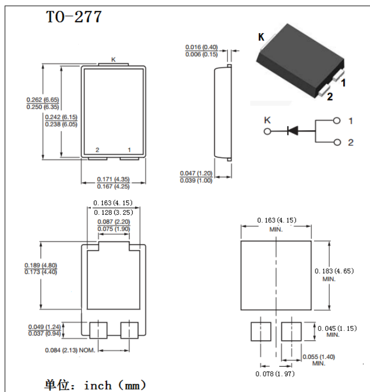
T0-277 封装外形图:
