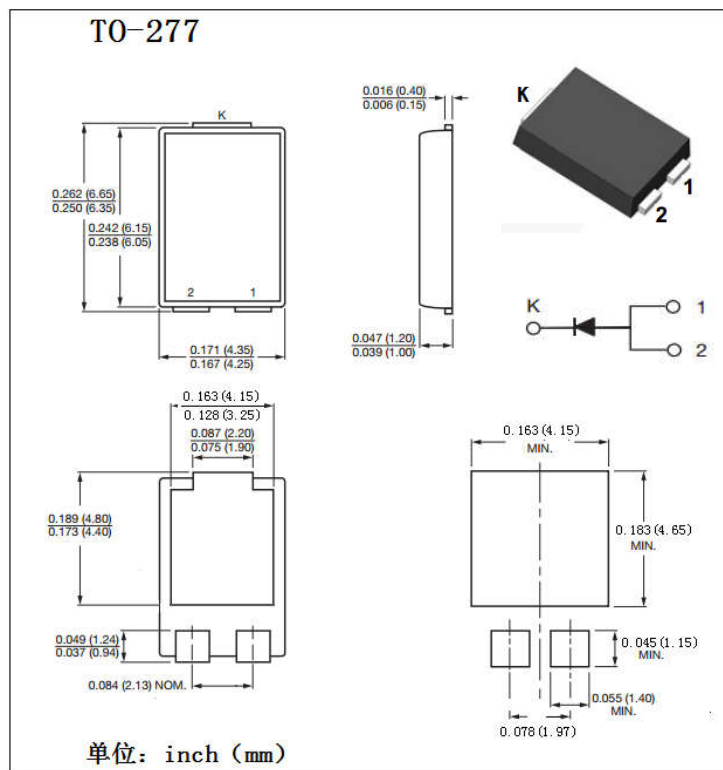
T0-277 封装外形图:
