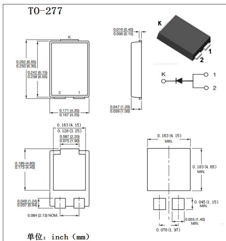
T0-277 封装外形图:
