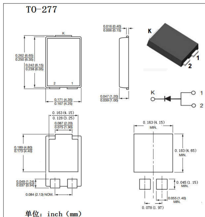
T0-277 封装外形图:
